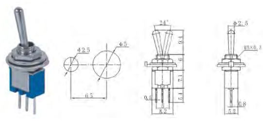
BTS-102-A2 ON-ON SPDT 3P
